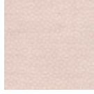
9-Patch
